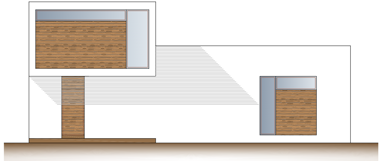
ALZADO NORTE
