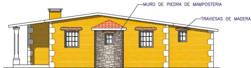
ALZADO NORESTE
