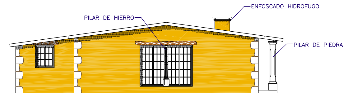
ALZADO SUROESTE
