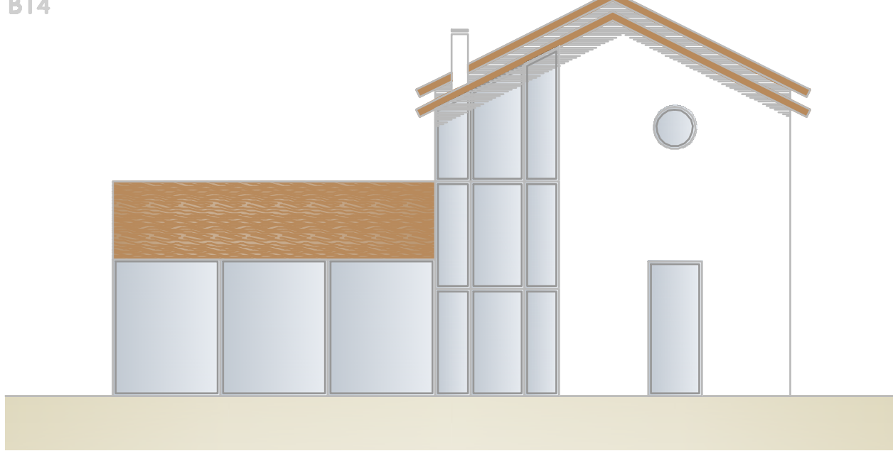
ALZADO SUR
