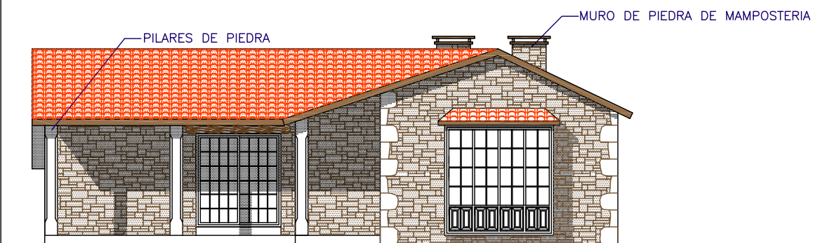
ALZADO SUR
