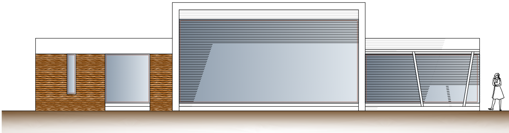
ALZADO SUR
