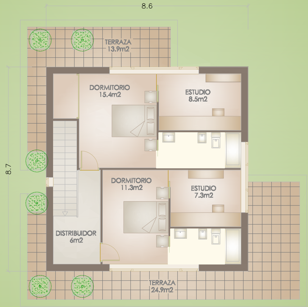
PLANTA PRIMERA
