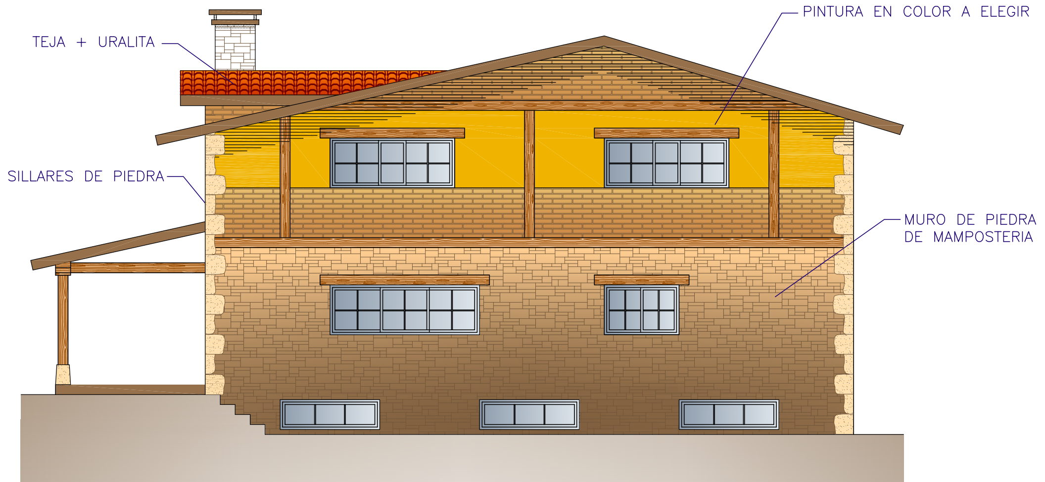
ALZADO ESTE
