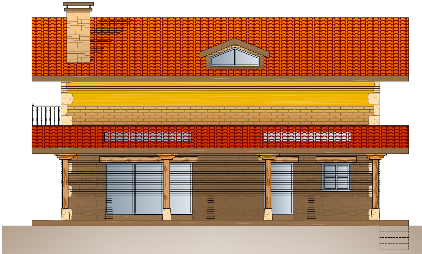
ALZADO SUR
