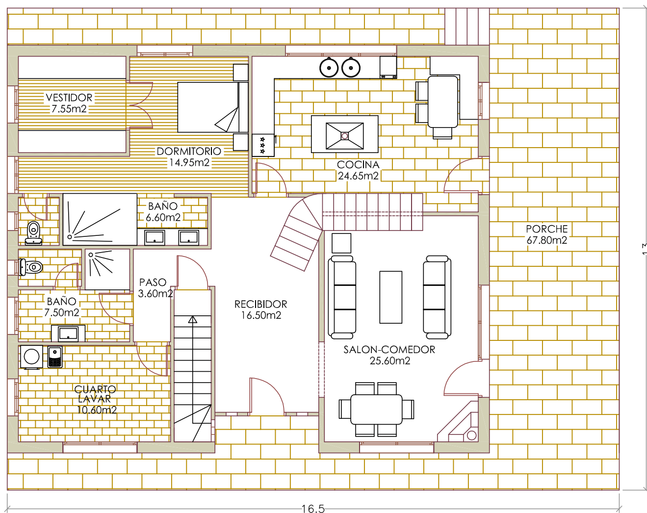
PLANTA BAJA
