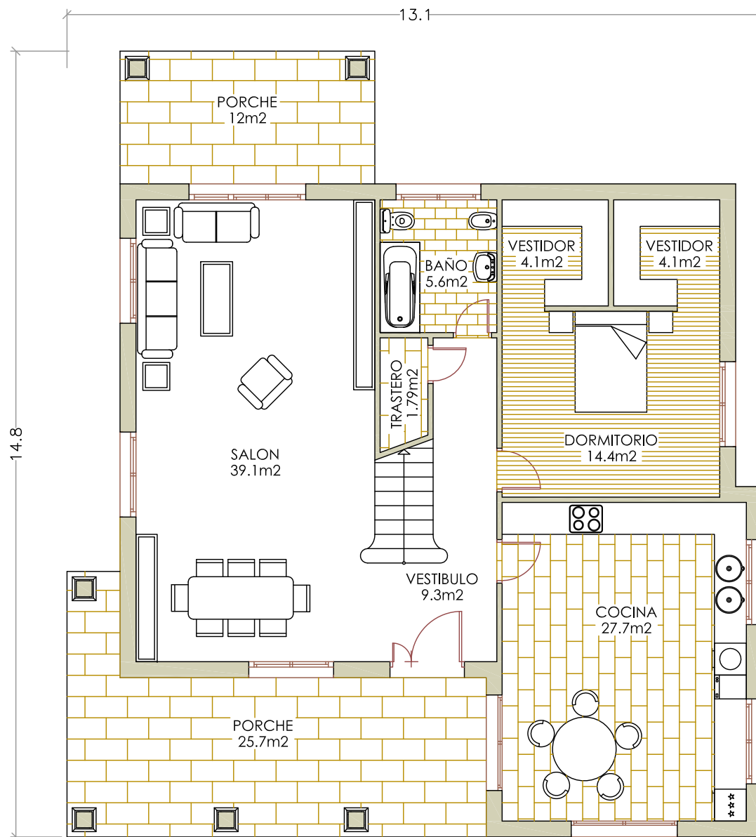
PLANTA BAJA
