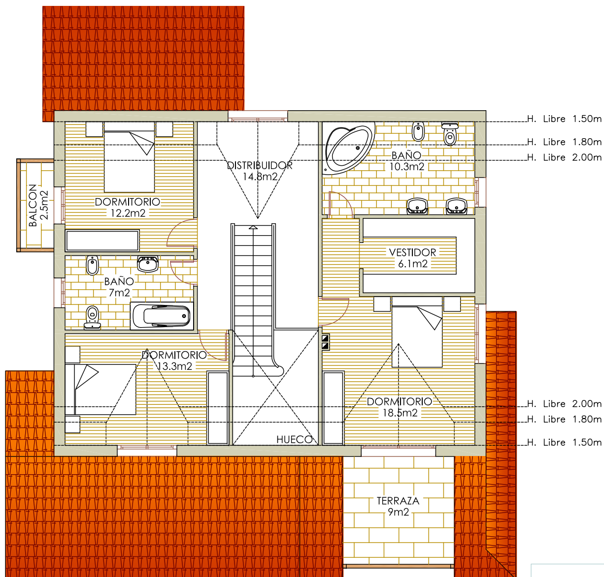
PLANTA BAJOCUBIERTA
