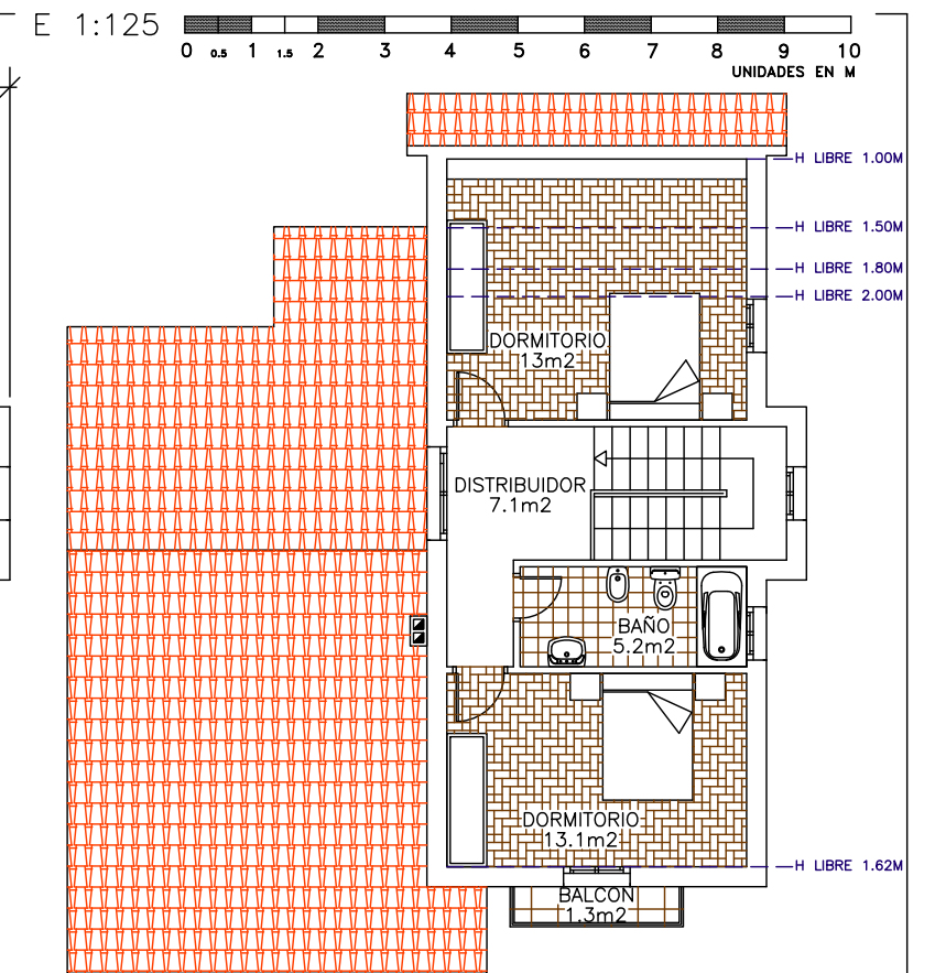
PLANTA BAJOCUBIERTA
