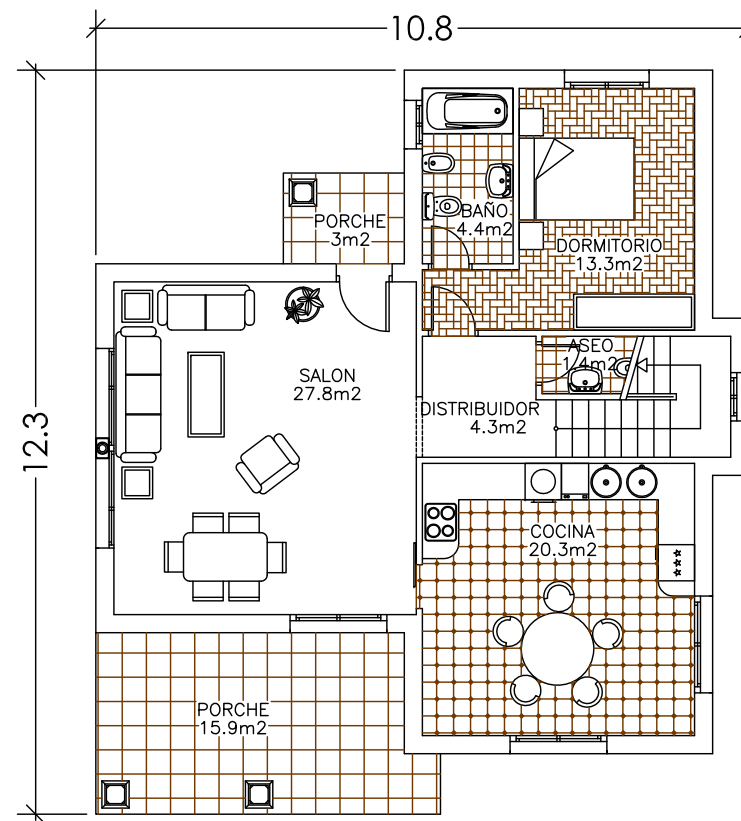
PLANTA BAJA
