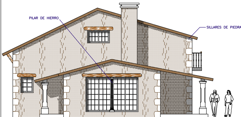
ALZADO OESTE
