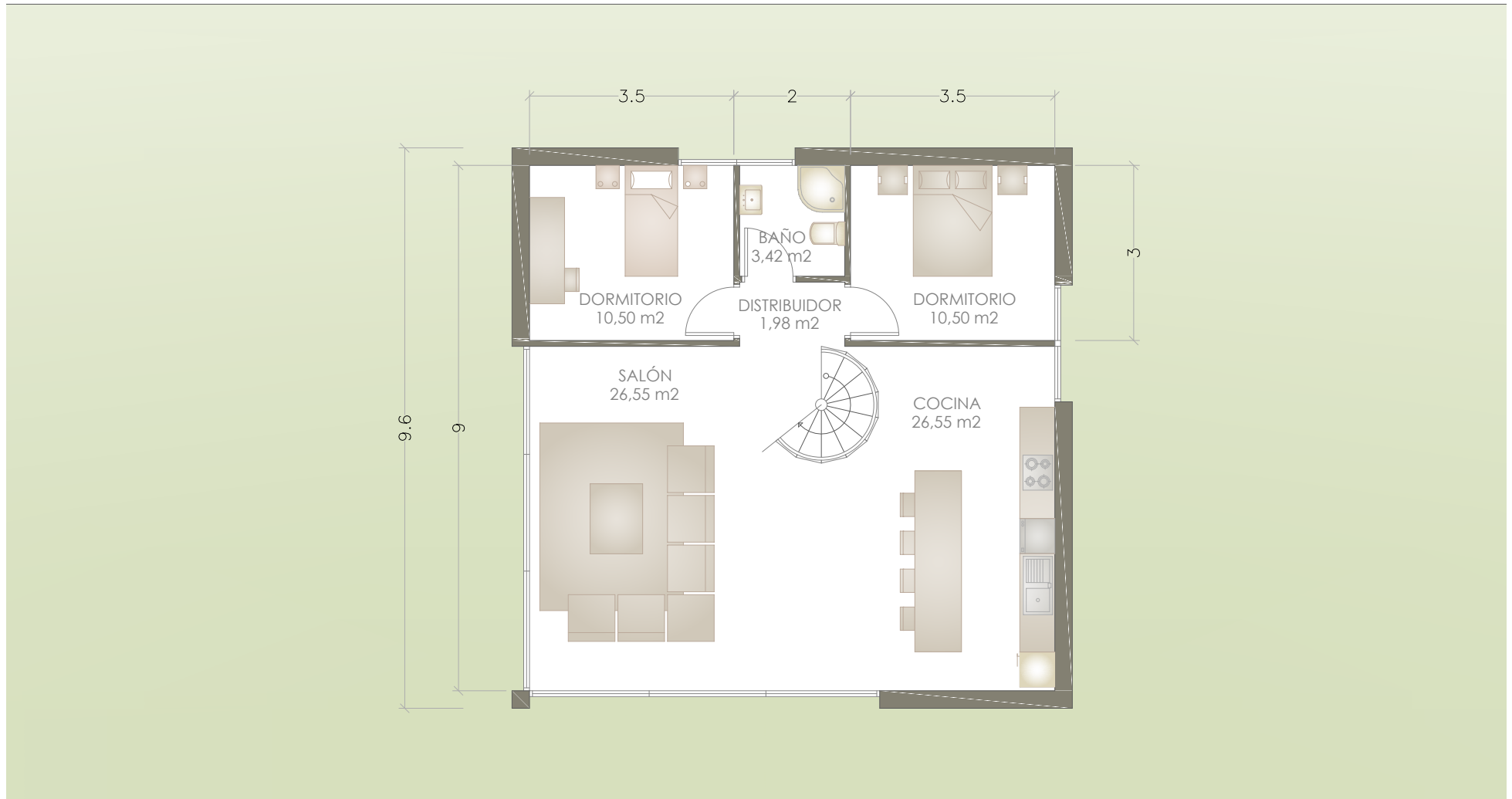
PLANTA BAJA
